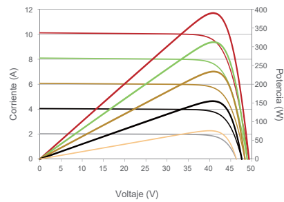
Curvas de corriente-voltaje y alimentación/voltaje (390W)
